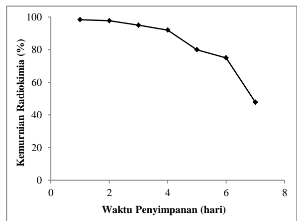
Gambar 4. Stabilitas Kemurnian Radiokimia Kit Cair Tetrofosmin pada Penyimpanan dalam Refrigerator
