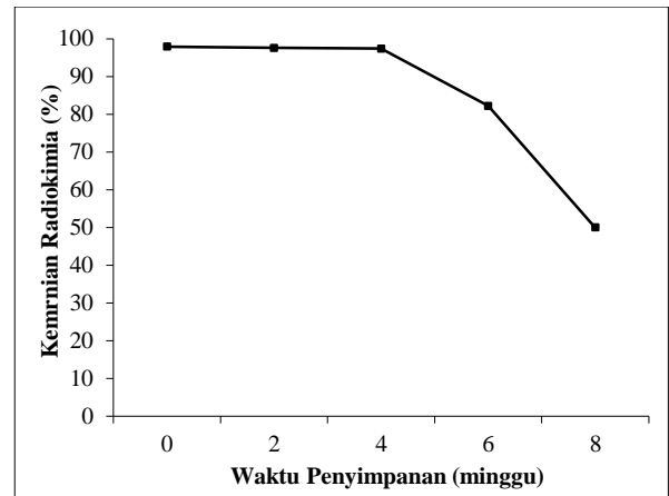
Gambar 3. Stabilitas Kemurnian Radiokimia Kit Cair Tetrofosmin penyimpanan dalam freezer.
